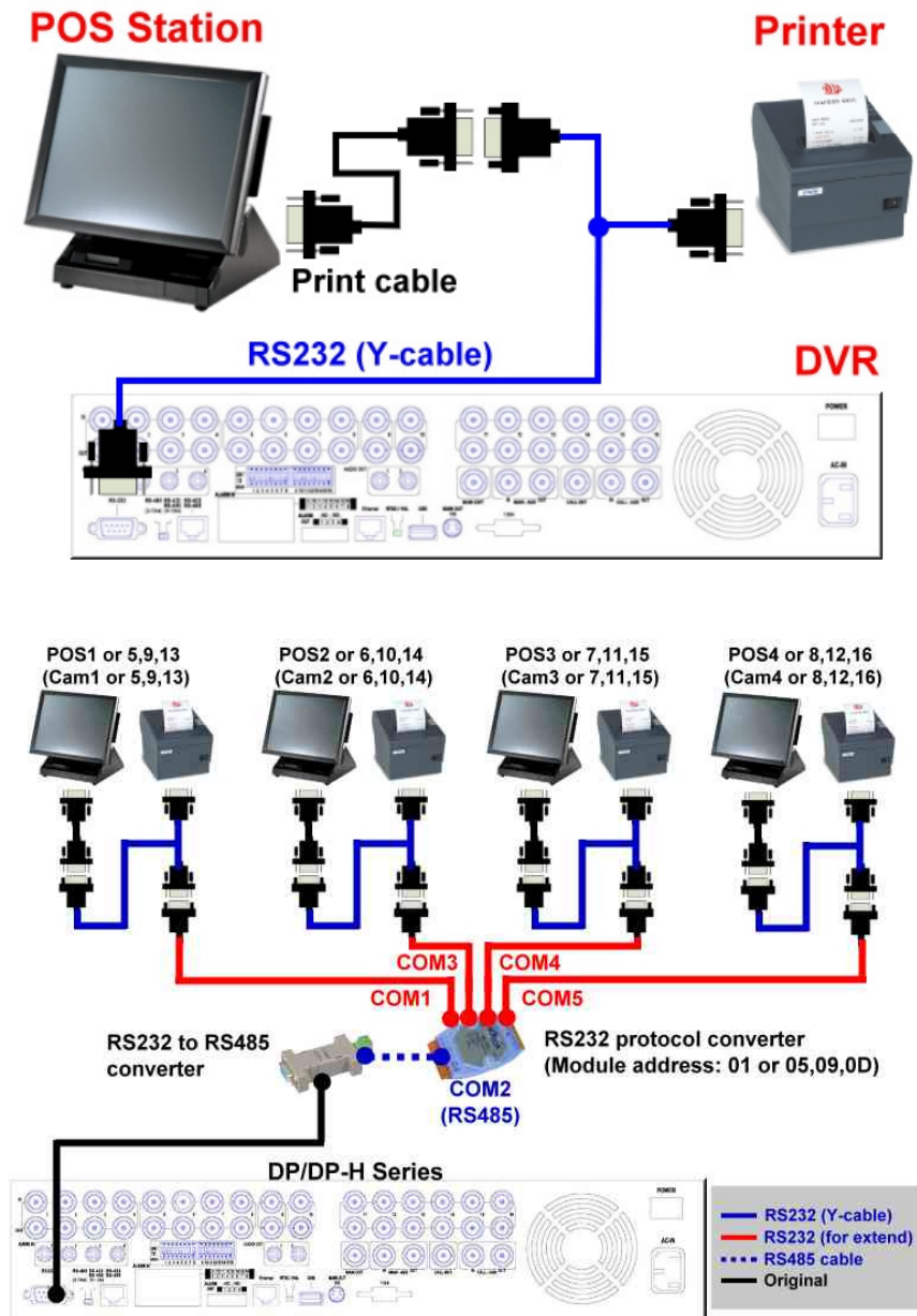
上圖：1 對 1；下圖：RS-232/多台 POS, 1 對多
